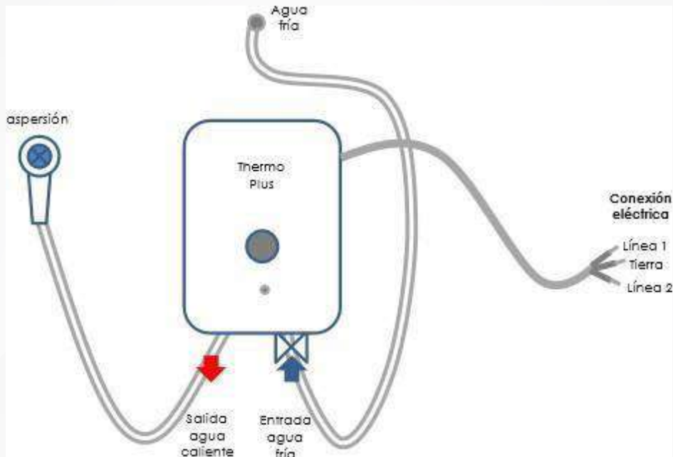
Figura N° 2 Conexión al Sistema de Agua
