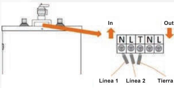
Figura N° 3 Conexión Eléctrica
