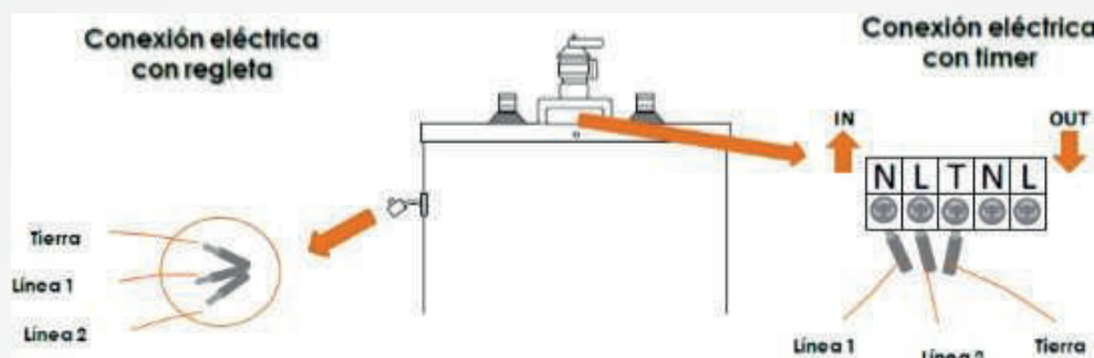
Figura N° 3 Conexión Eléctrica
