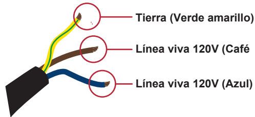
Figura N° 3 Conexión Eléctrica
