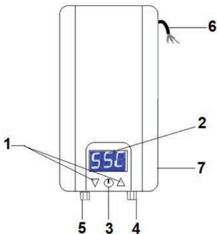
Figura N°1 Partes del THERMO MASTER PRO
