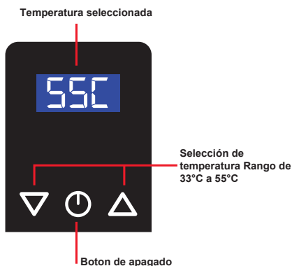
Figura N° 4 Funcionamiento del Thermo Master
