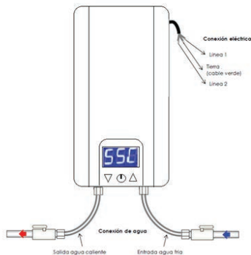
Figura N° 2 Conexión al Sistema de Agua
