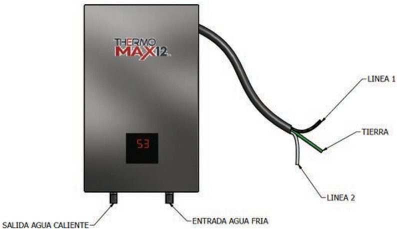
Figura N° 2 Conexión al Sistema de Agua
