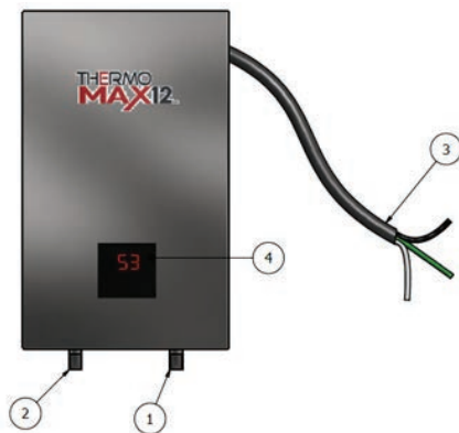
Figura N°1 Partes del THERMO MAX
