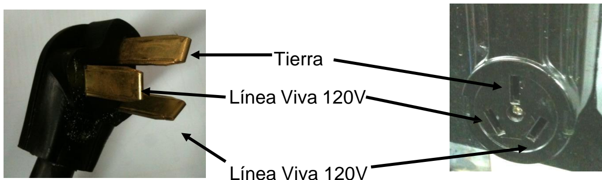
Figura N° 3 Conexión Eléctrica
