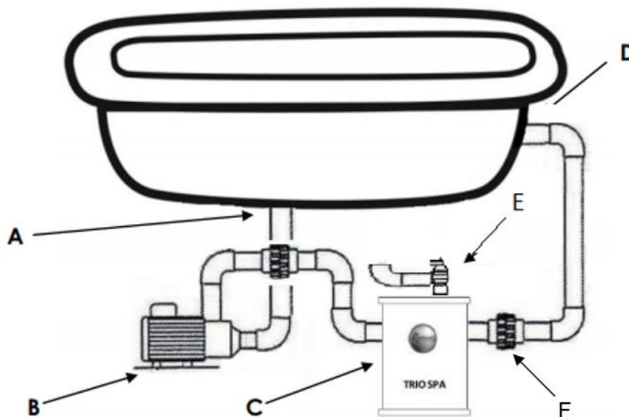
Figura N°2 Diagrama de Instalación
