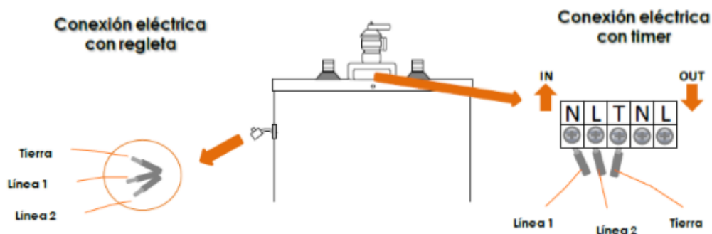
Figura N° 3 Conexión Eléctrica
