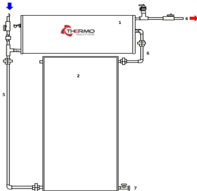
Figura N°1 Partes del THERMO SOLAR
