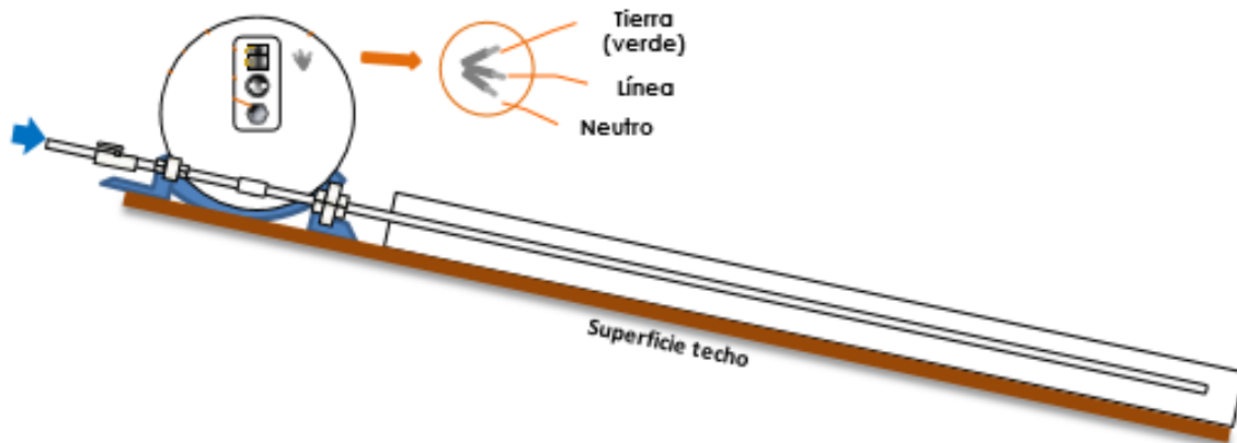
Figura N° 3 Conexión Eléctrica
