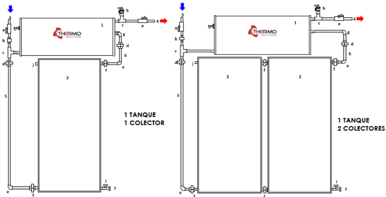
Figura N° 2 Conexión al Sistema de Agua
