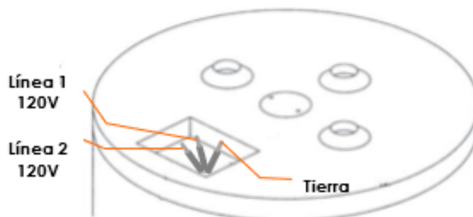
Figura N° 3 Conexión Eléctrica
