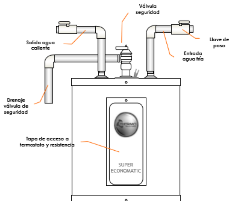
Figura N° 2 Conexión al Sistema de Agua
