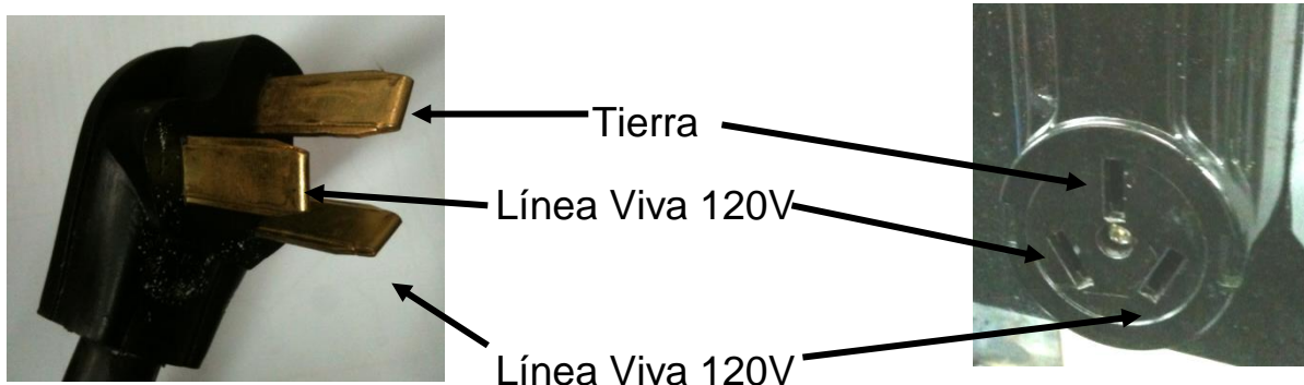
Figura N° 3 Conexión Eléctrica
